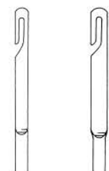
ST22-505-25 ST22-505-30 Ø 2.5 mm Ø 3.0 mm
